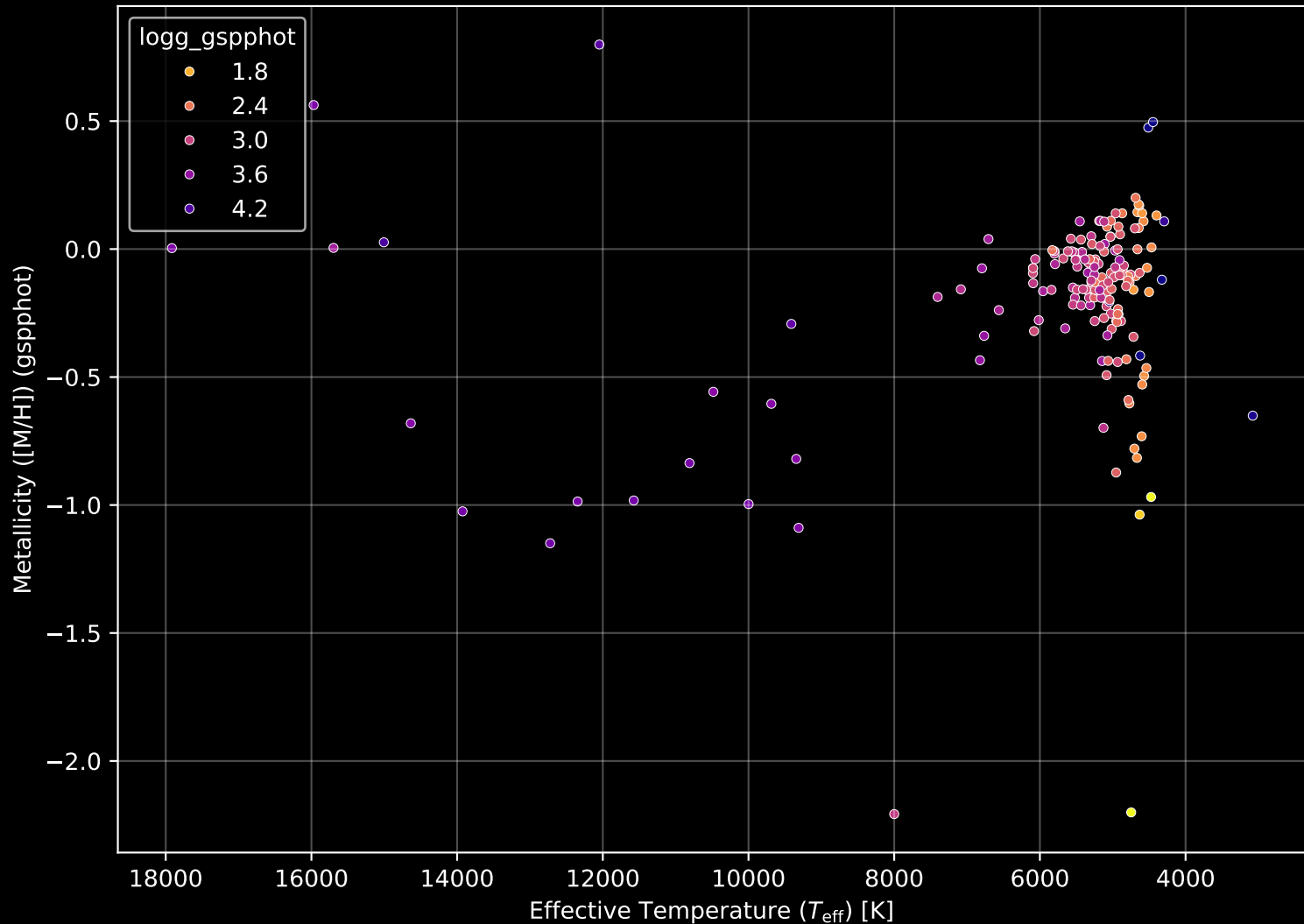
APOGEE DR17 Field: [191-04] Stellar Population Parameters (n= 176)
